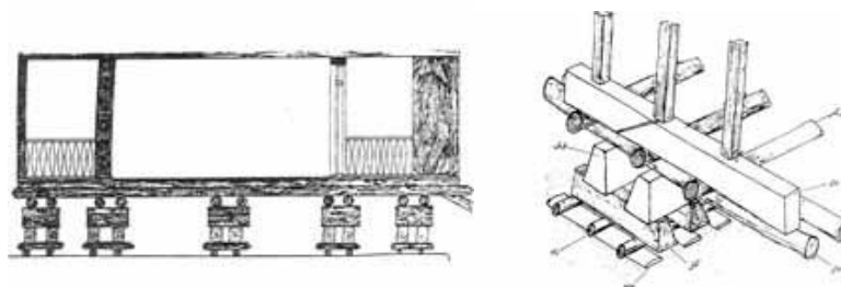
شکل ۳ ایجاد کرسی برای جدا کردن ساختمان از کف
