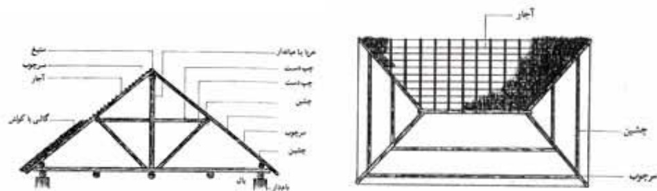
شکل ۲ اجزای سقف شیروانی در شیوه ی سنتی آن
