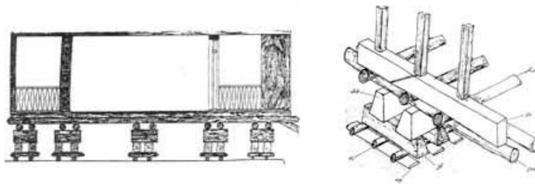
شکل 3 ایجاد کرسی برای جدا کردن ساختمان از کف
